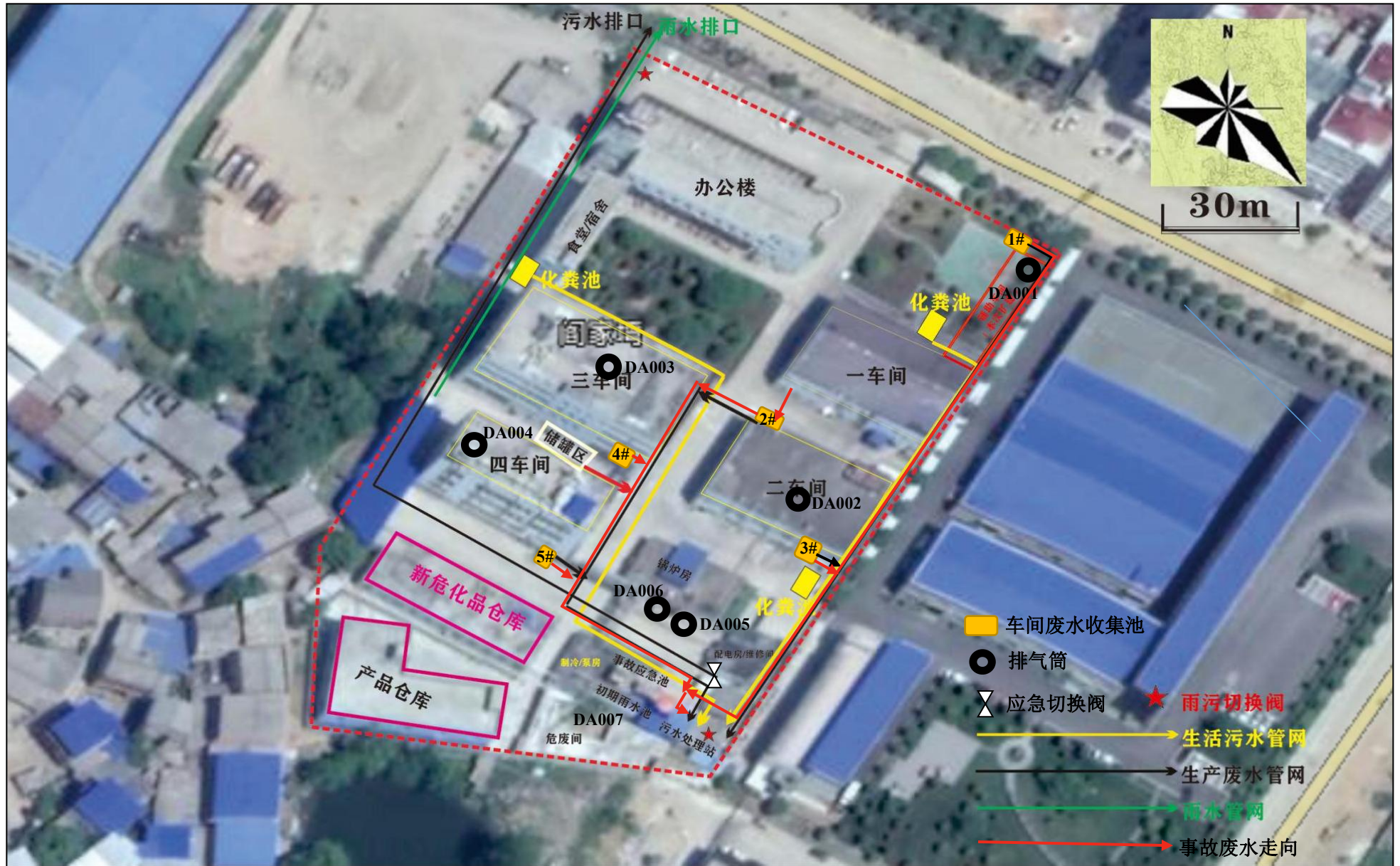
附图 5 项目环保设施及雨污管网布置图
